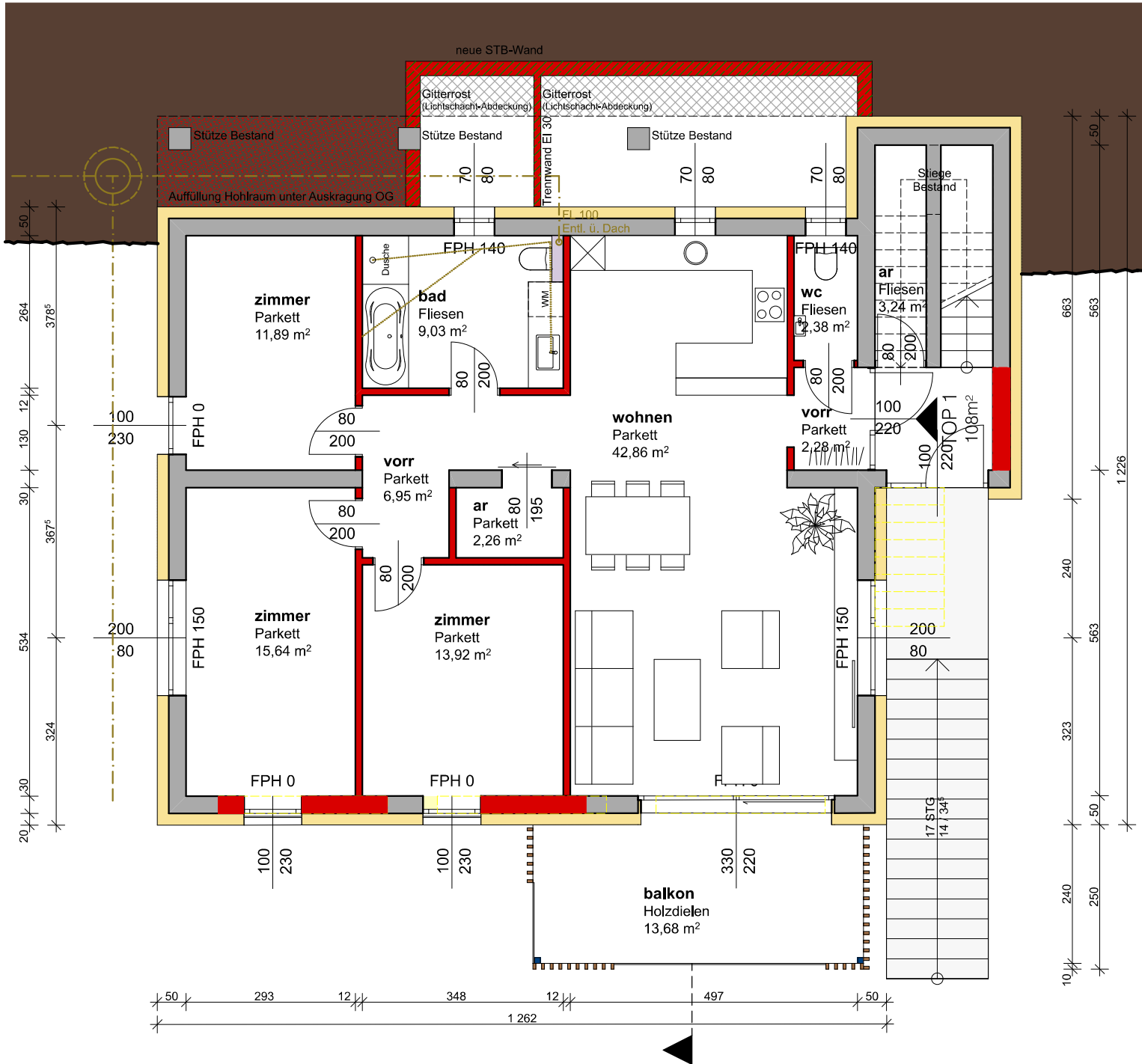
Erdgeschoß
