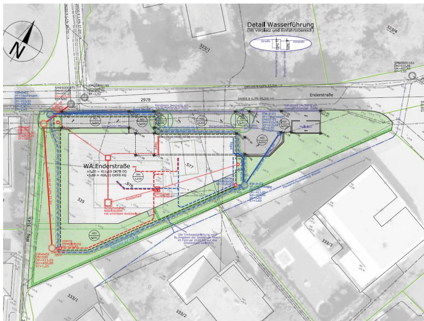
Auszug Entwässerungsplanung
