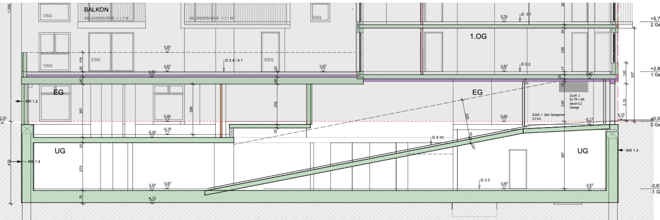
SCHNITT 1 HOF RAMPE GARAGE
