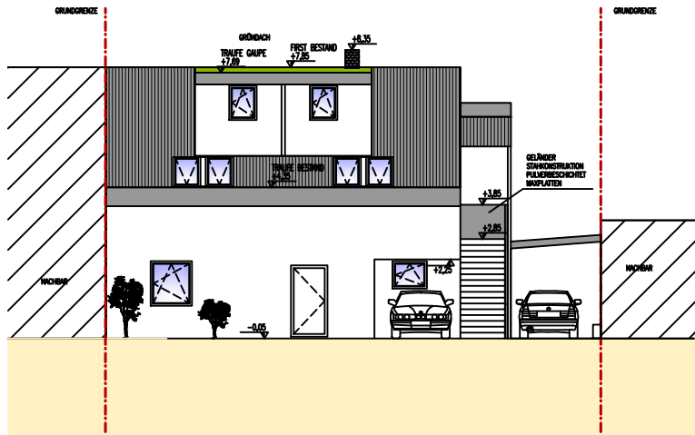
ANSICHT WEST M 1:200
