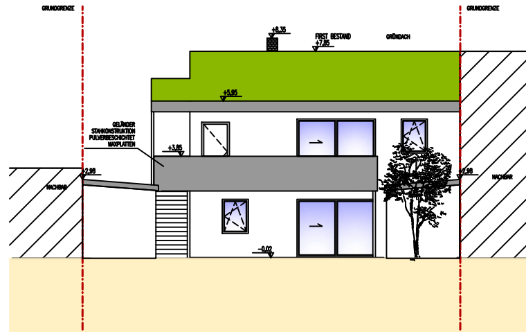
ANSICHT OST M 1:200
