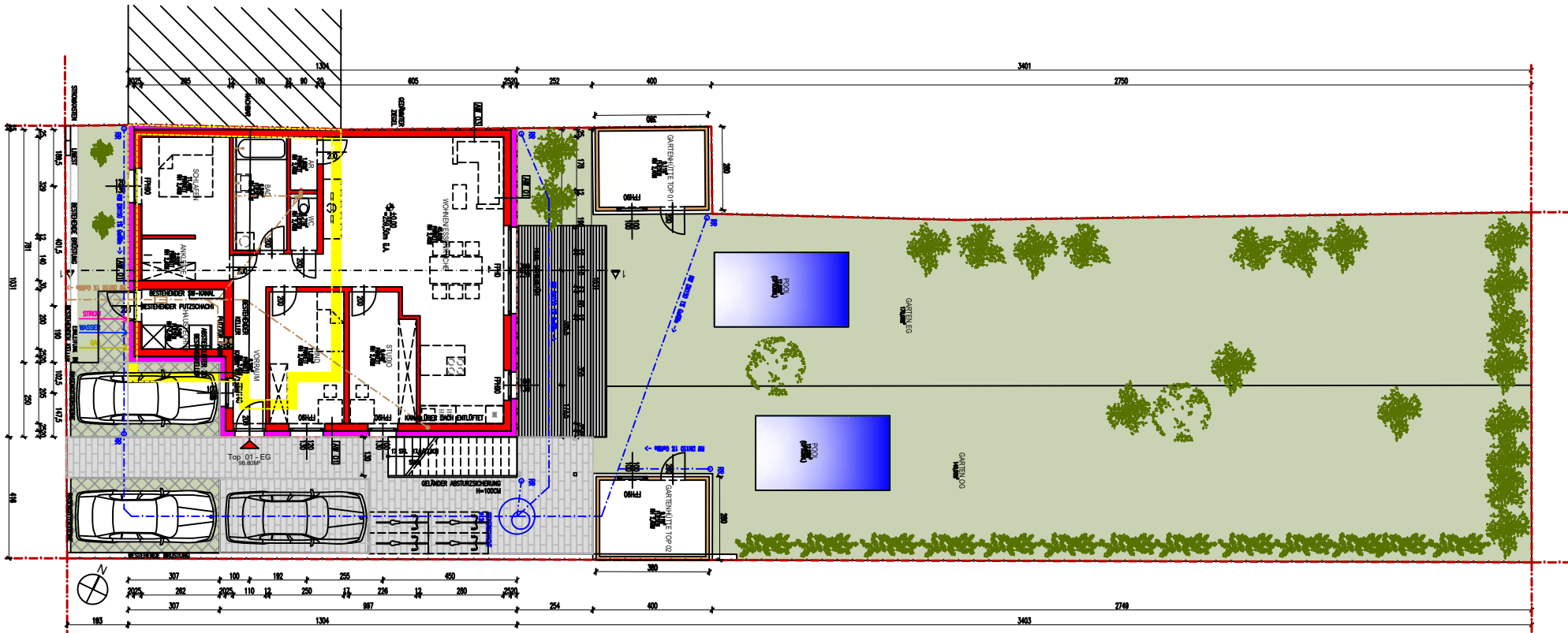
GRUNDRISS EG M 1:200
