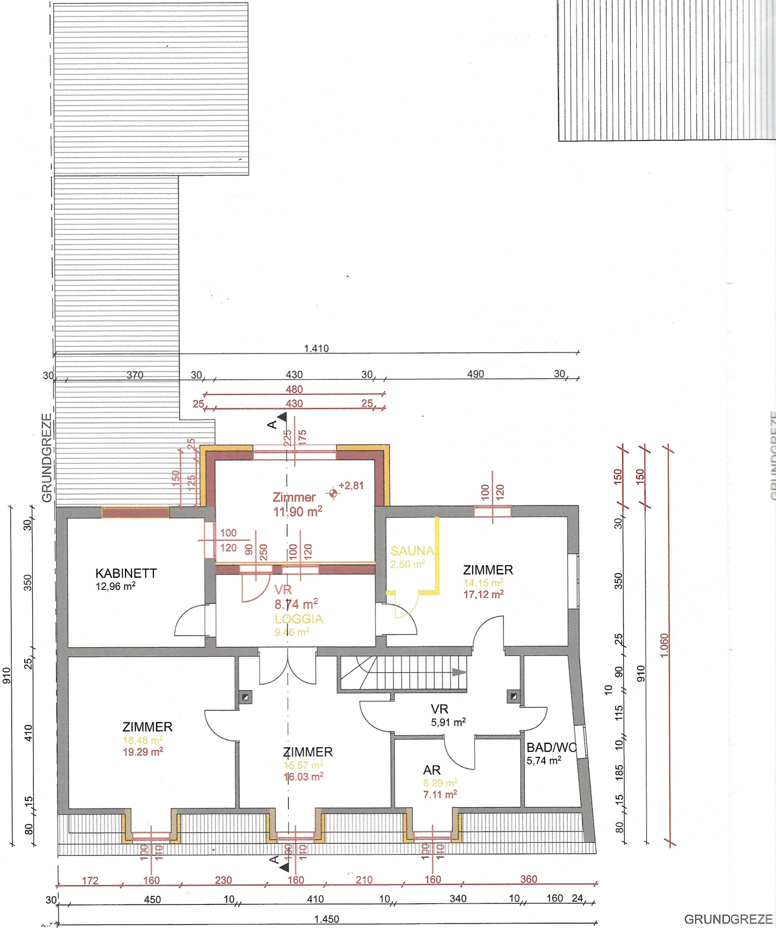
OBERGESCHOSS 1:100
