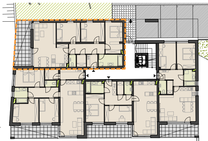
Lageübersicht Erdgeschoß
