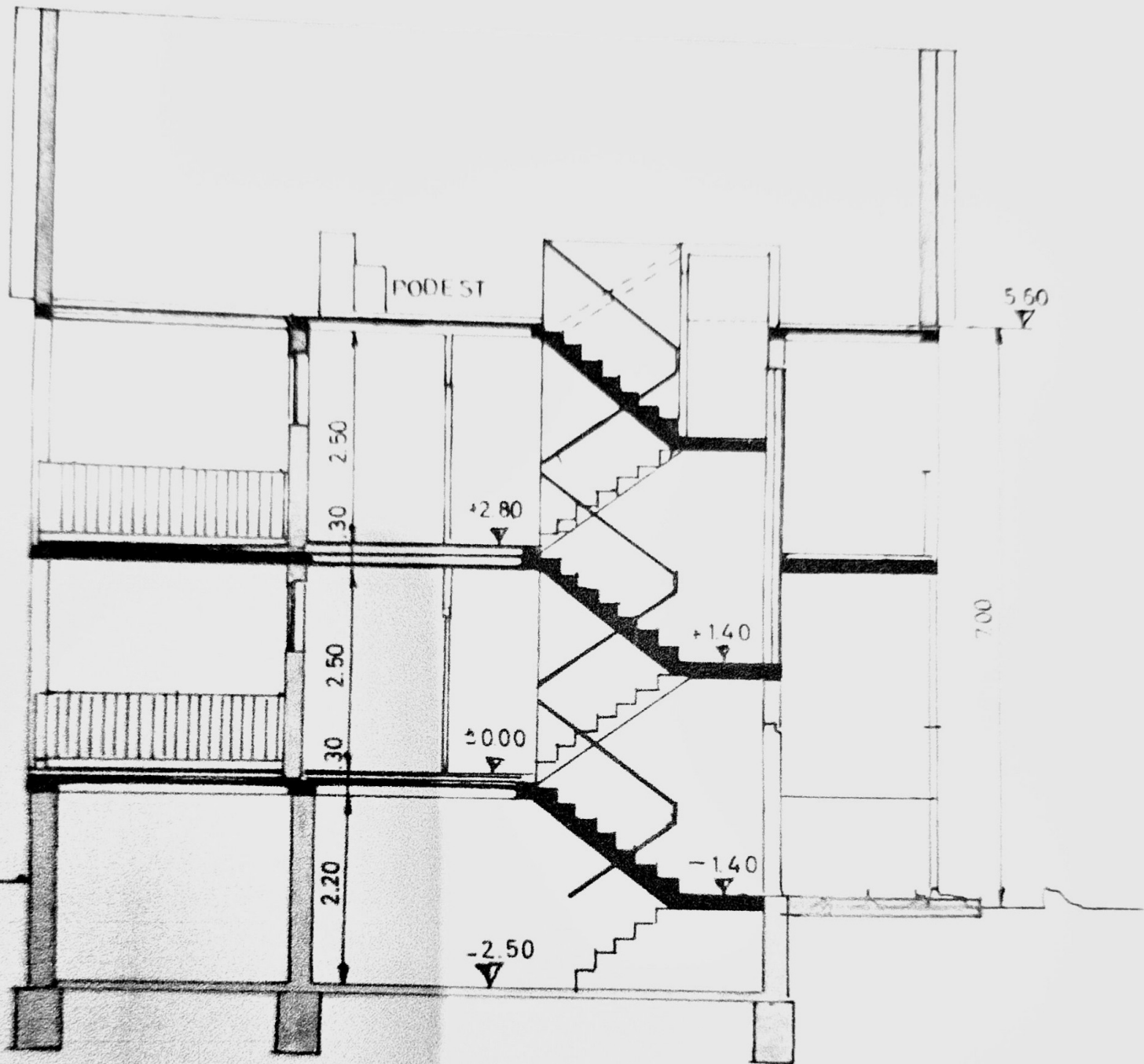
N ORD - SÜD SCHNITT
