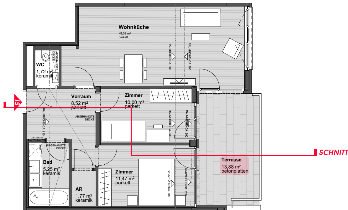
Grundriss | M 1:100
