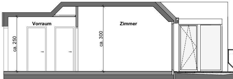
Schnitt | M 1:100
