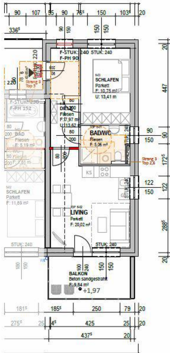
1. OBERGESCHOSS M 1:100
