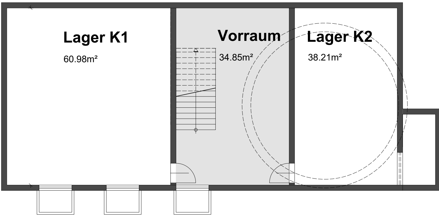
Grundriss Kellergeschoss 1:100
