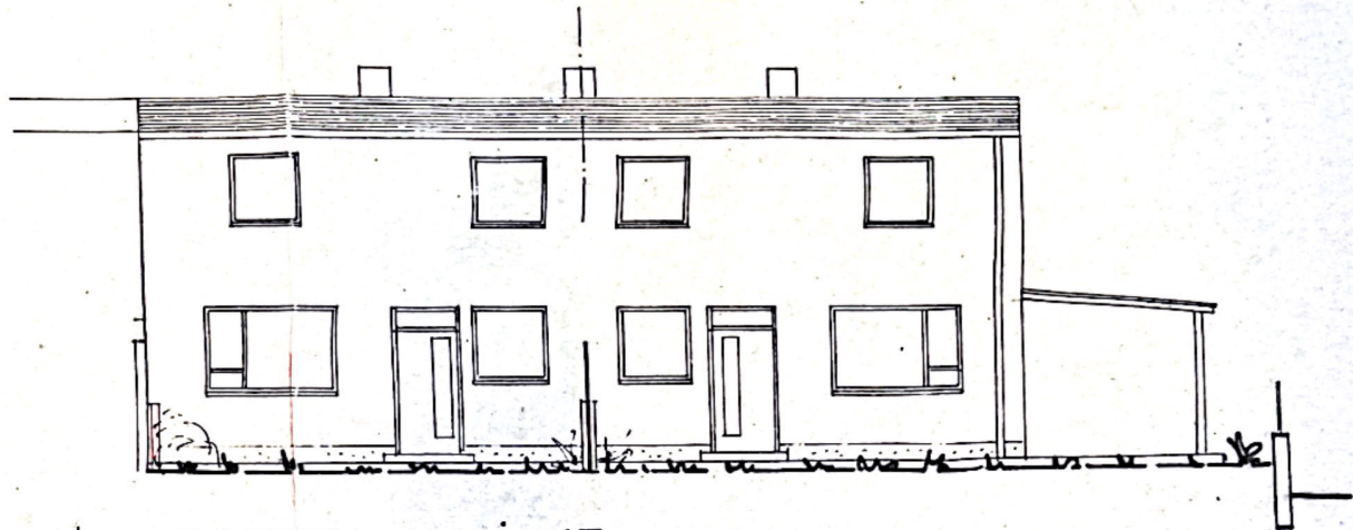
GARTEN-ANSICHT
