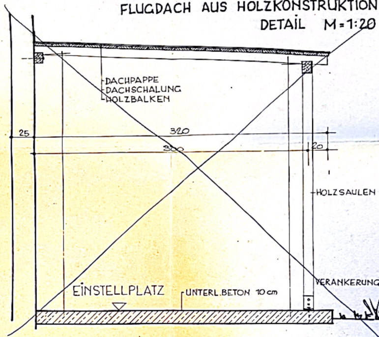
WEG - ANSICHT
