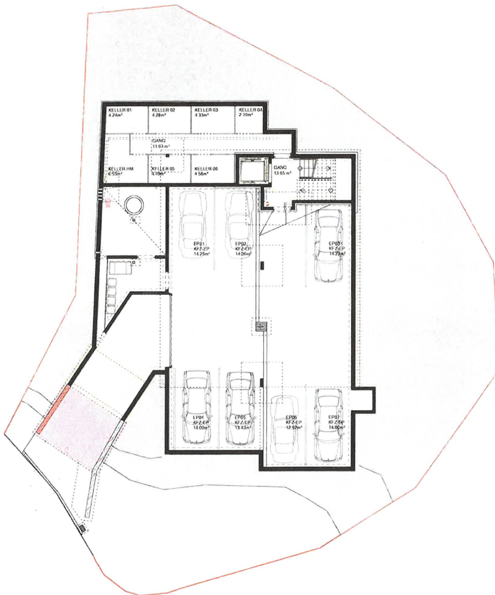
Untergeschoss M: 1: 200
