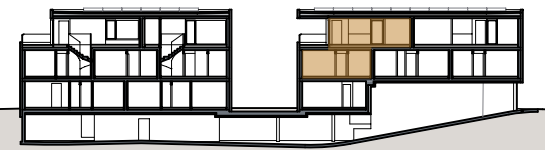
SCHNITT
