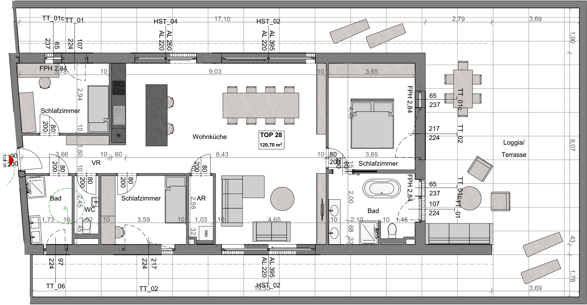
VERKAUFSPLAN TOP 28 1:100
