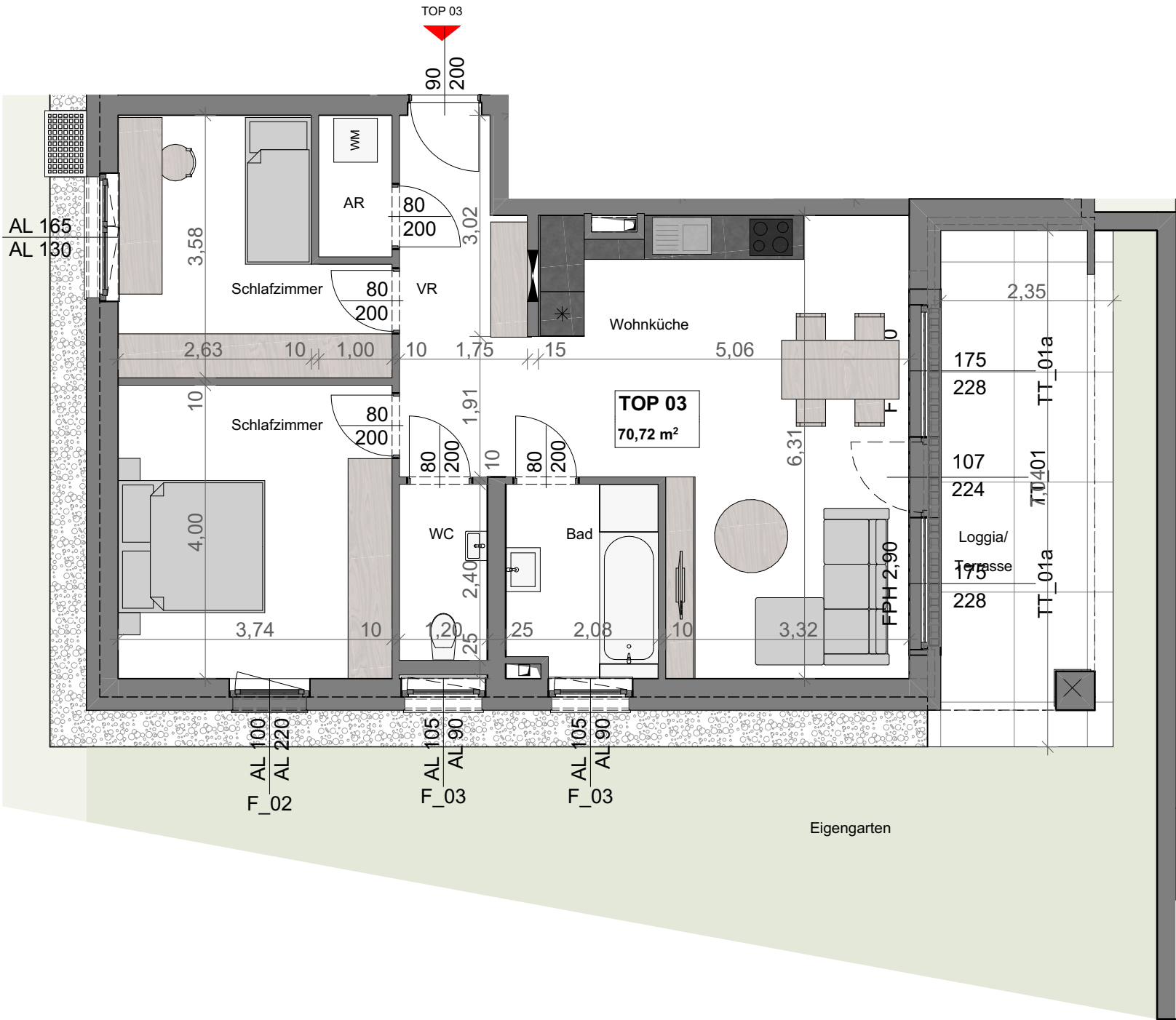
VERKAUFSPLAN TOP 03 1:75
