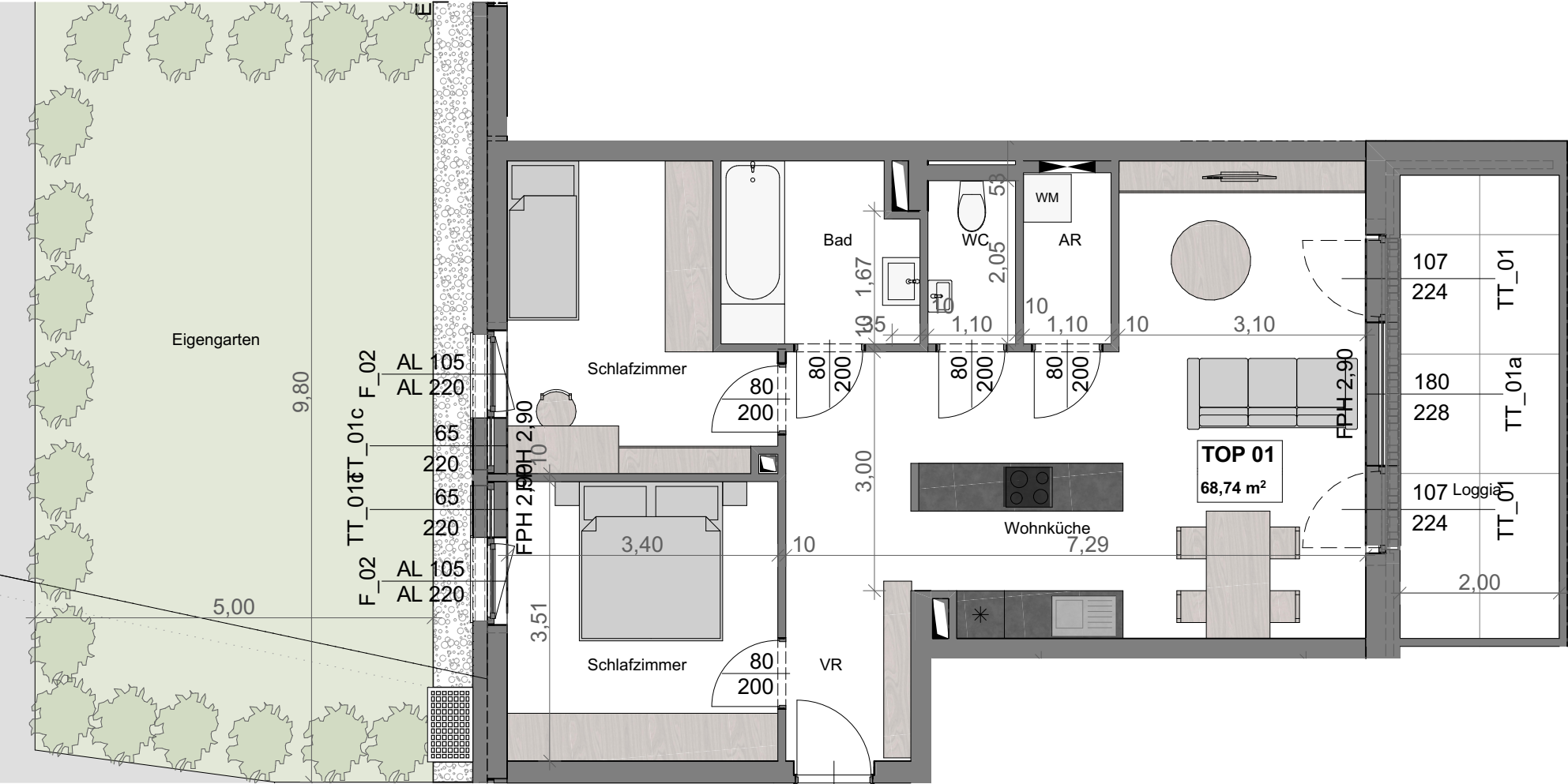
VERKAUFSPLAN TOP 01 1:75
