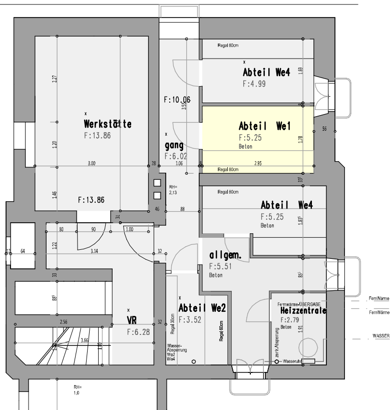
GRUNDRISS Kellerabteil
