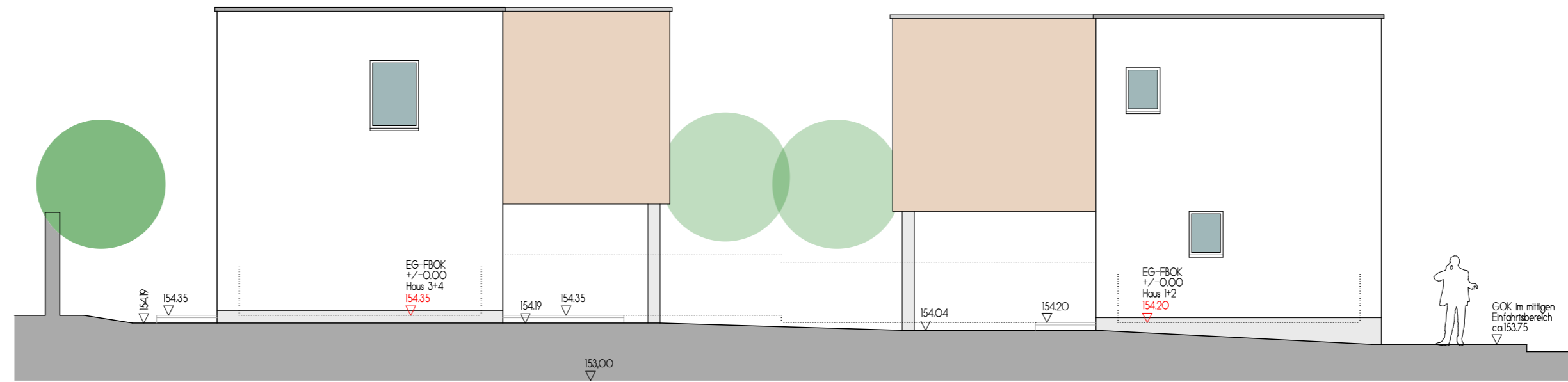
Schnitt C-C in Einfahrtsrichtung
