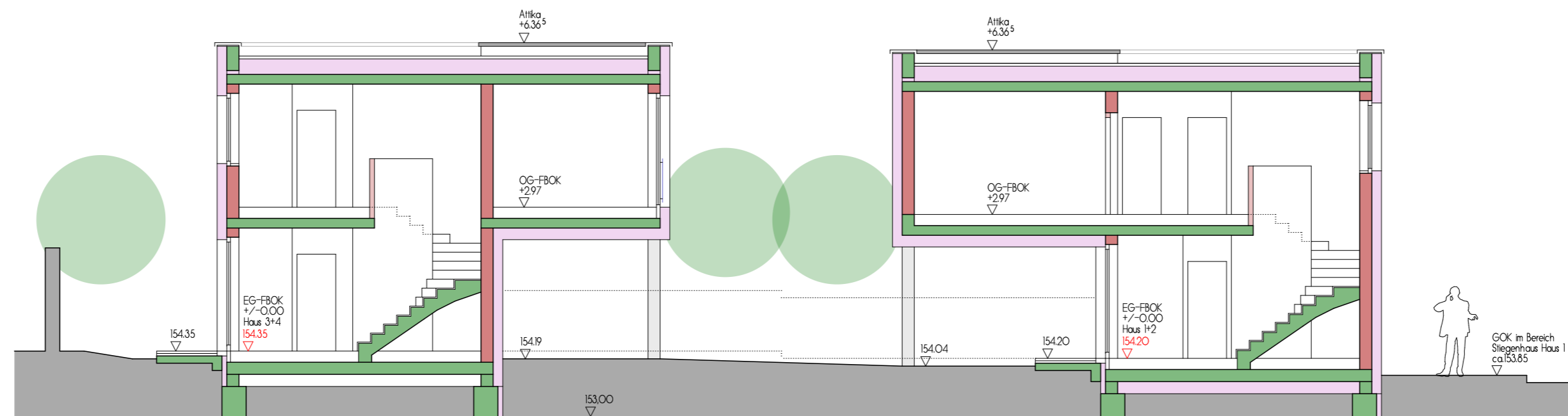
Schnitt B-B durch Stiegenhäuser
