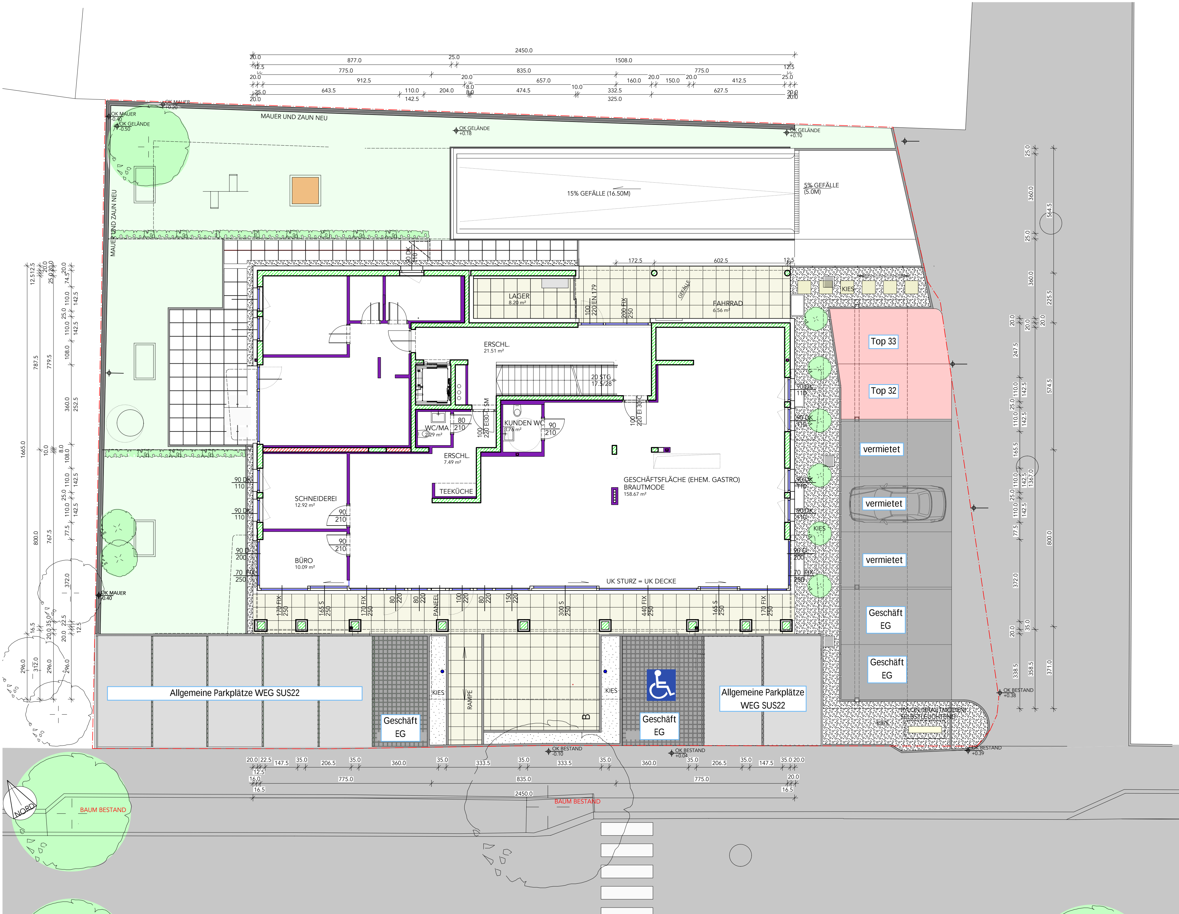
GRUNDRISS ERDGESCHOSS M1:100
