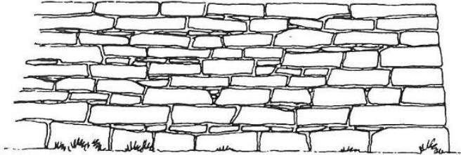
Lagerhaftes Bruchsteinmauerwerk
