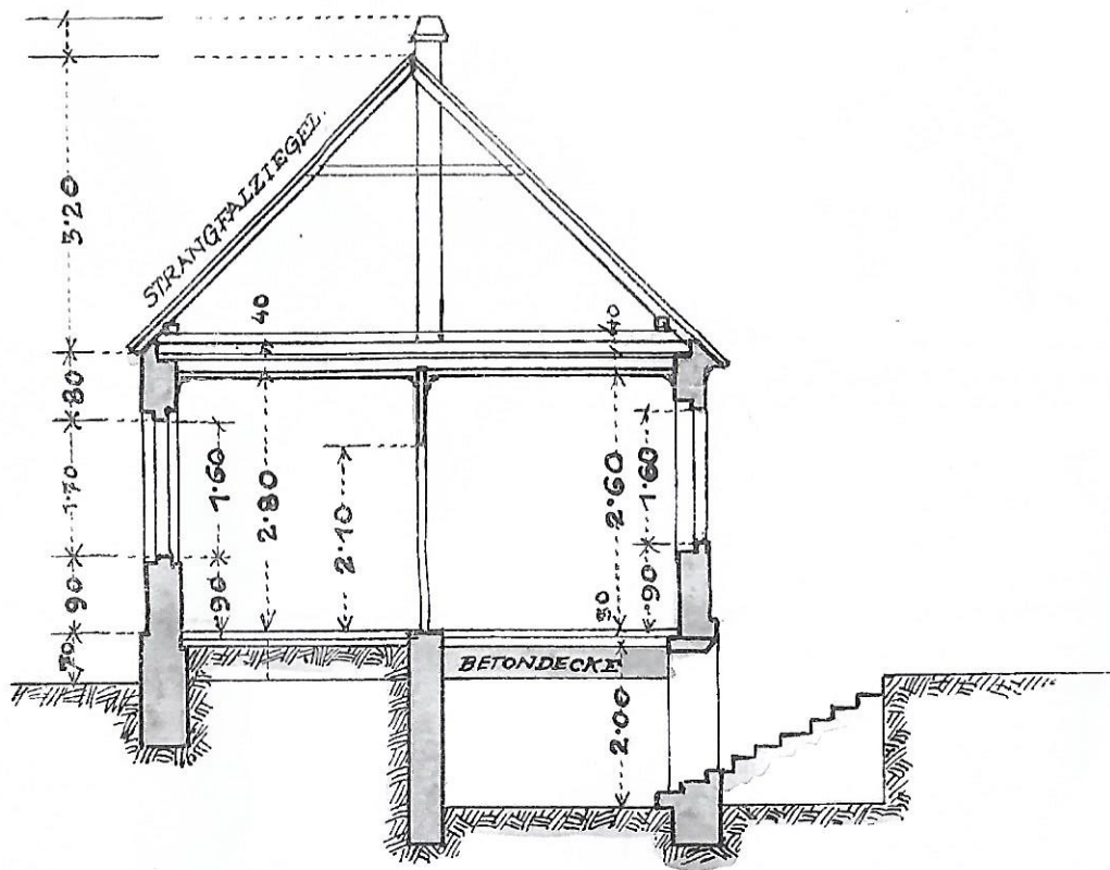
SCHNITT: II
