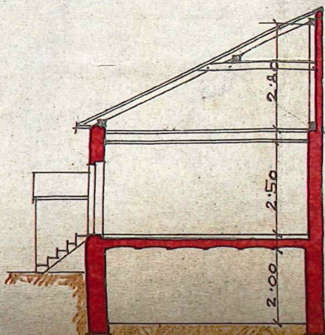
SCHNITT
