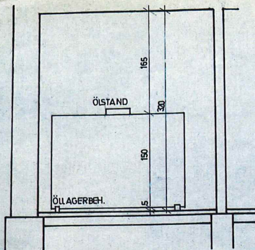
SCHNITT M 1/50
