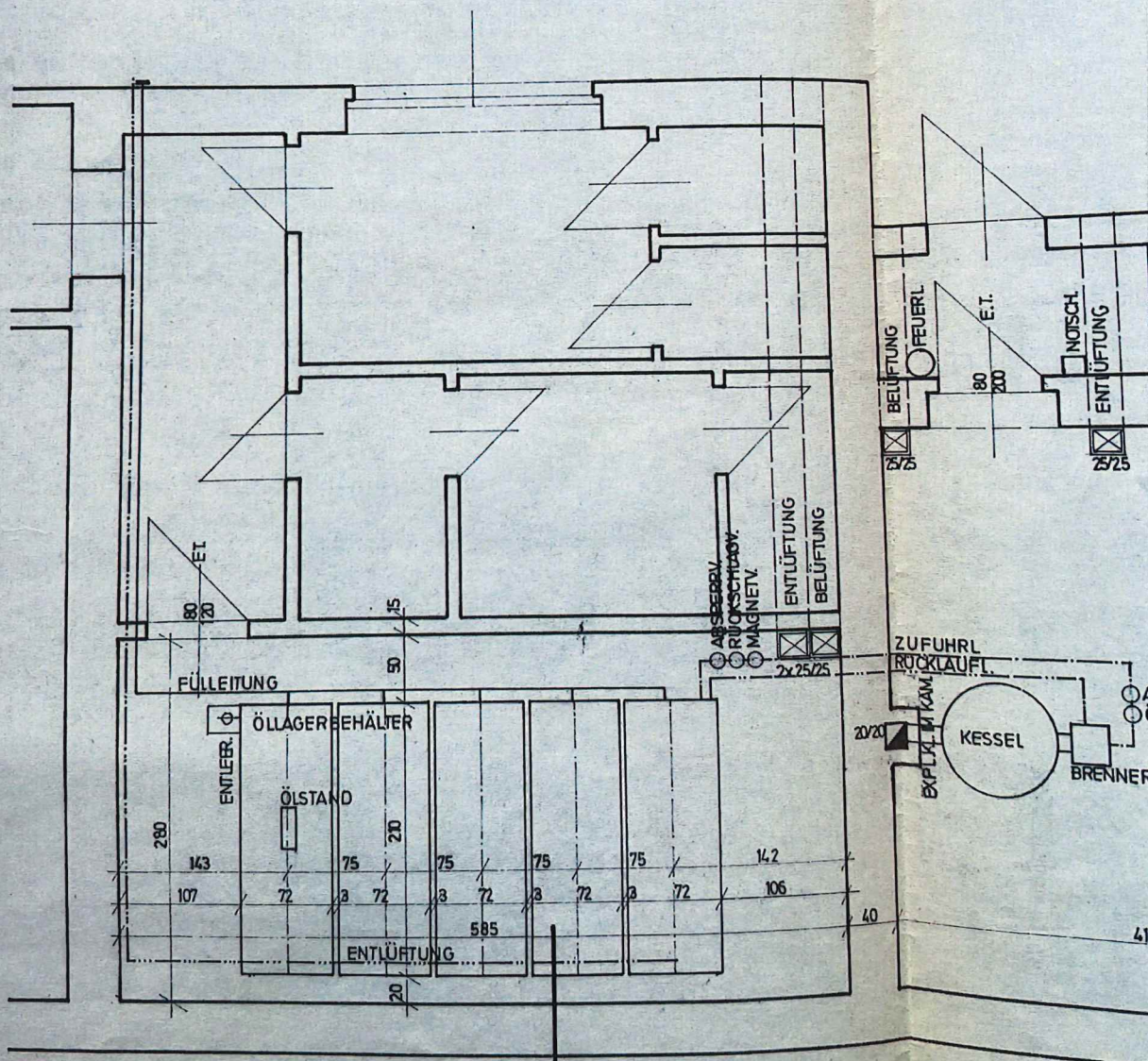
GRUNDRISS M 1/50
