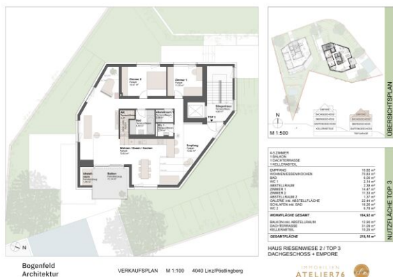
Grundriss Variante 4 Zimmer
