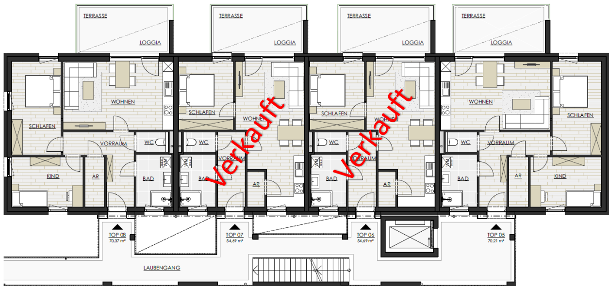
Übersichtsplan Obergeschoss Haus Nord
