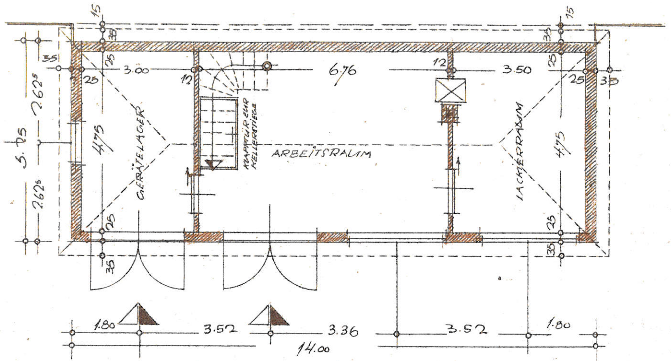
ERDGESCHOSS M. 1:100
