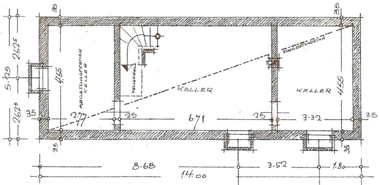
KELLER M. 1:100
