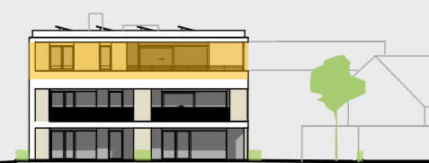
südwest ansicht
